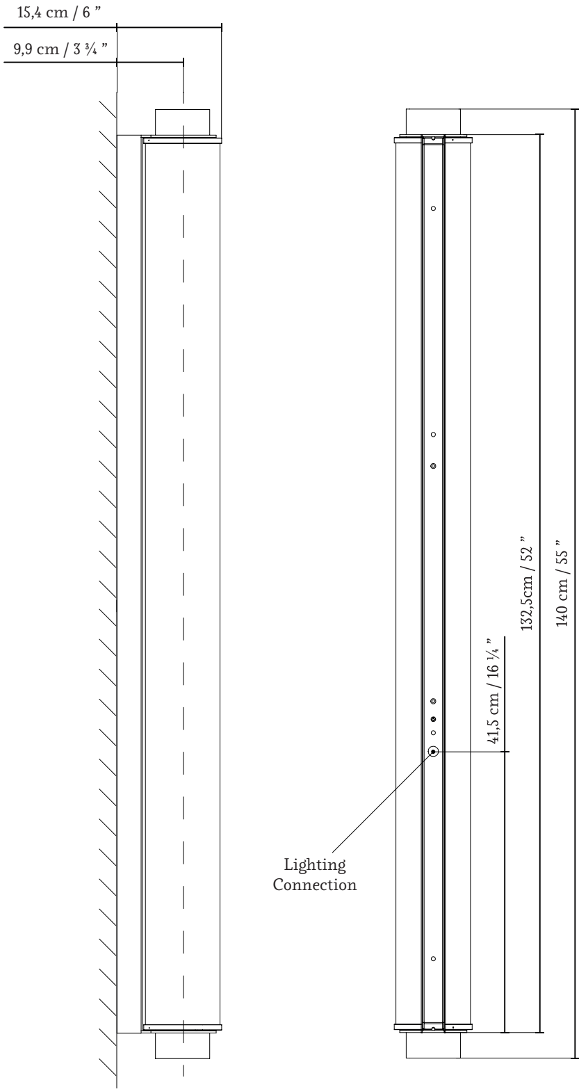
1. Dimensiones generales de la luminaria
