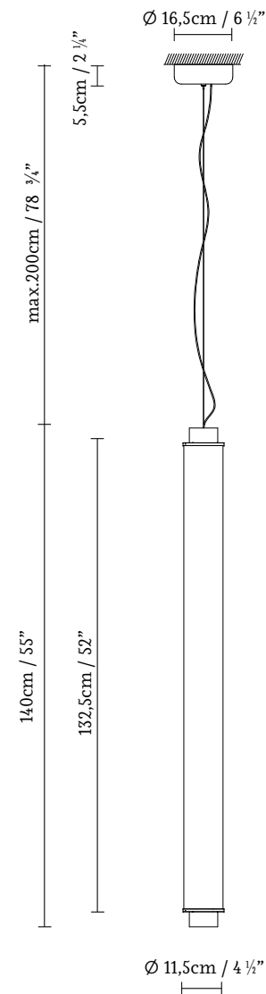
SLIM SKIN SV1400
