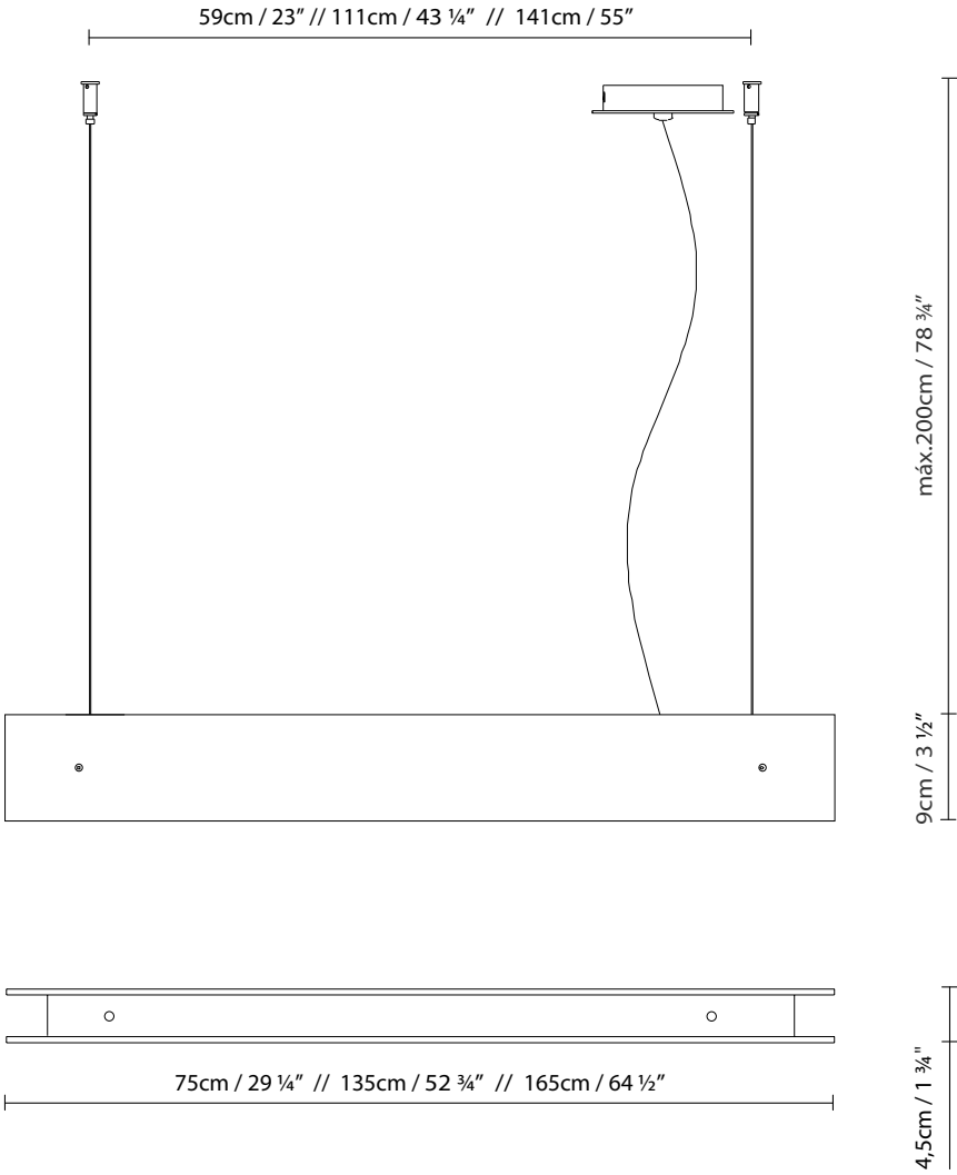
MARC S 70 2L / MARC S 130 2L / MARC S 160 2L
