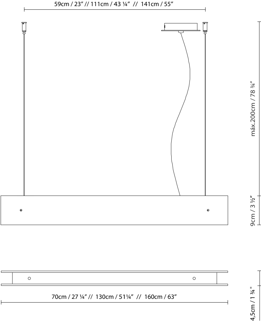
MARC S 70 1L / MARC S 130 1L / MARC S 160 1L
